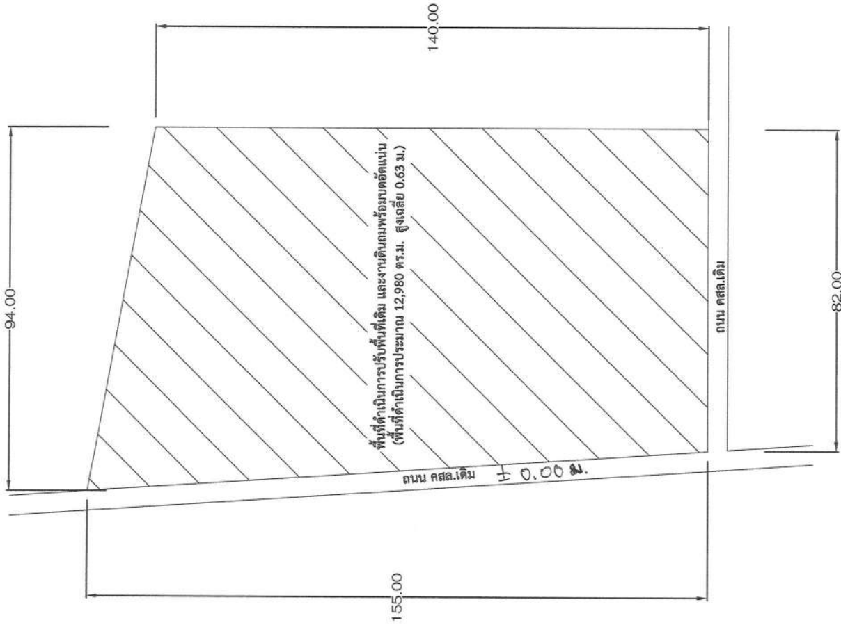
แผนผังบริเวณที่ตั้งโครงการพอสังเซป Not to Scale
